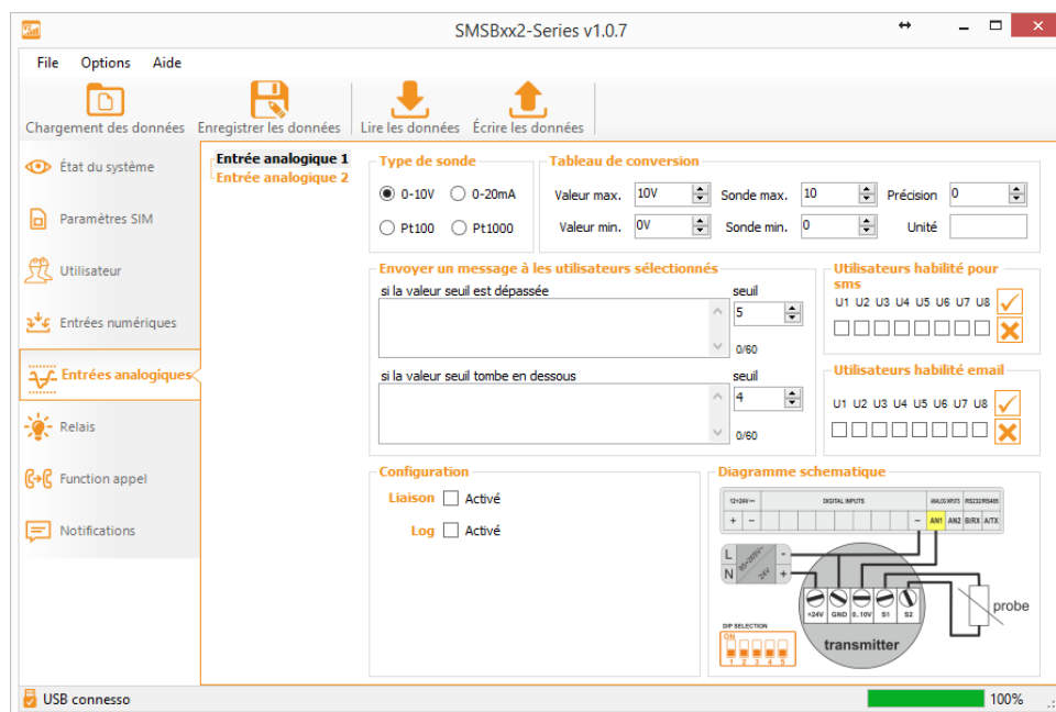
Image 5: Entrées analogiques
