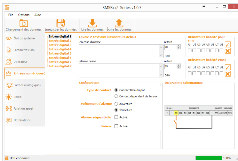
Image 4: Entrées numériques
